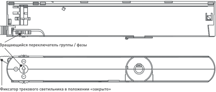
Рис. 3. Расположение фиксатора и переключателя на источнике питания
