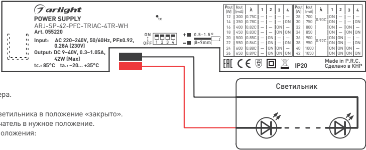
Рис. 2. Подключение светильника к источнику питания
