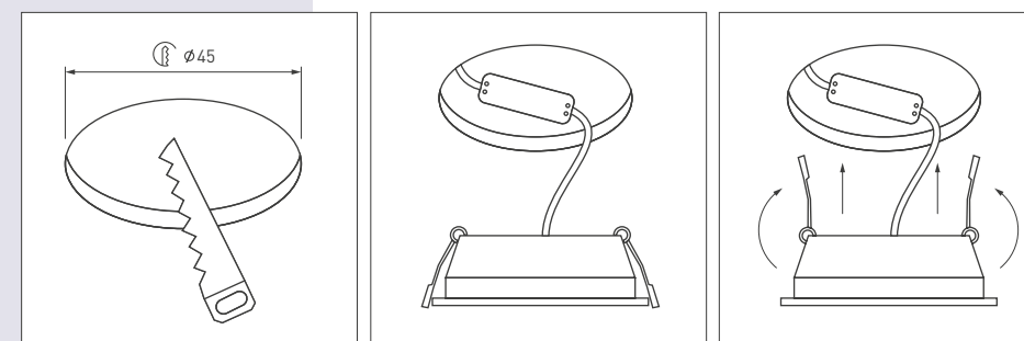
Схема установки и подключения
