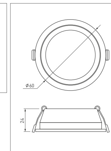
Конструктивный чертеж
