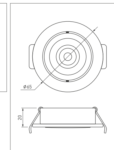
Конструктивный чертеж
