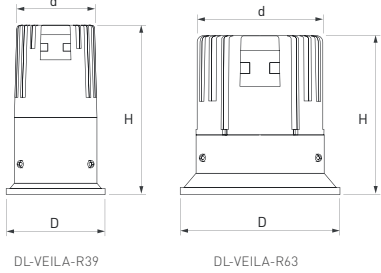
Рис. 1. Габаритный чертеж
