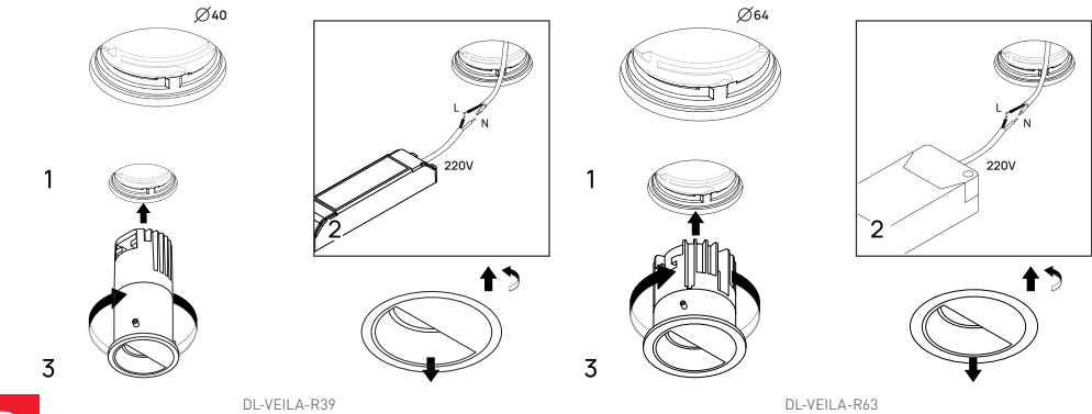
Рис. 2. Схема монтажа
